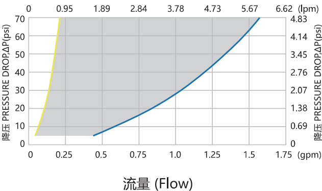
五通路系列 水流 (Five channel series Water Flow)
