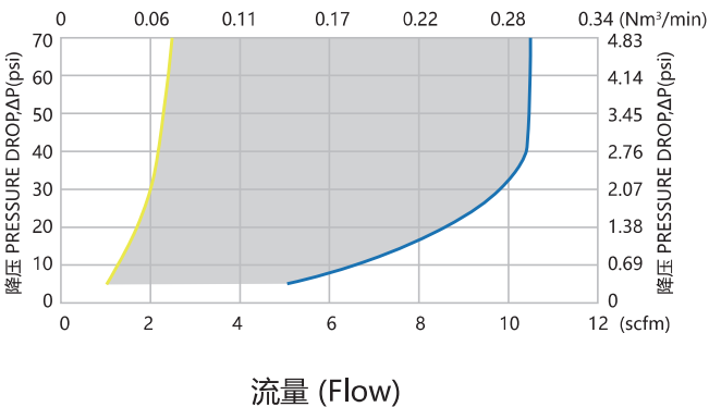
五通路系列 气流 (Five channel series airflow)
